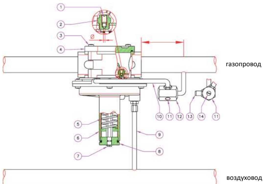
Рис. 4 Соотношение газ/воздух = 2:1 - 10:1
