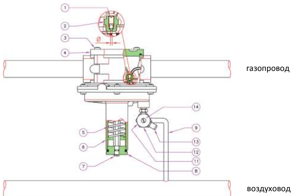
Рис. 3 Соотношение газ/воздух = 1:2 - 1:10
